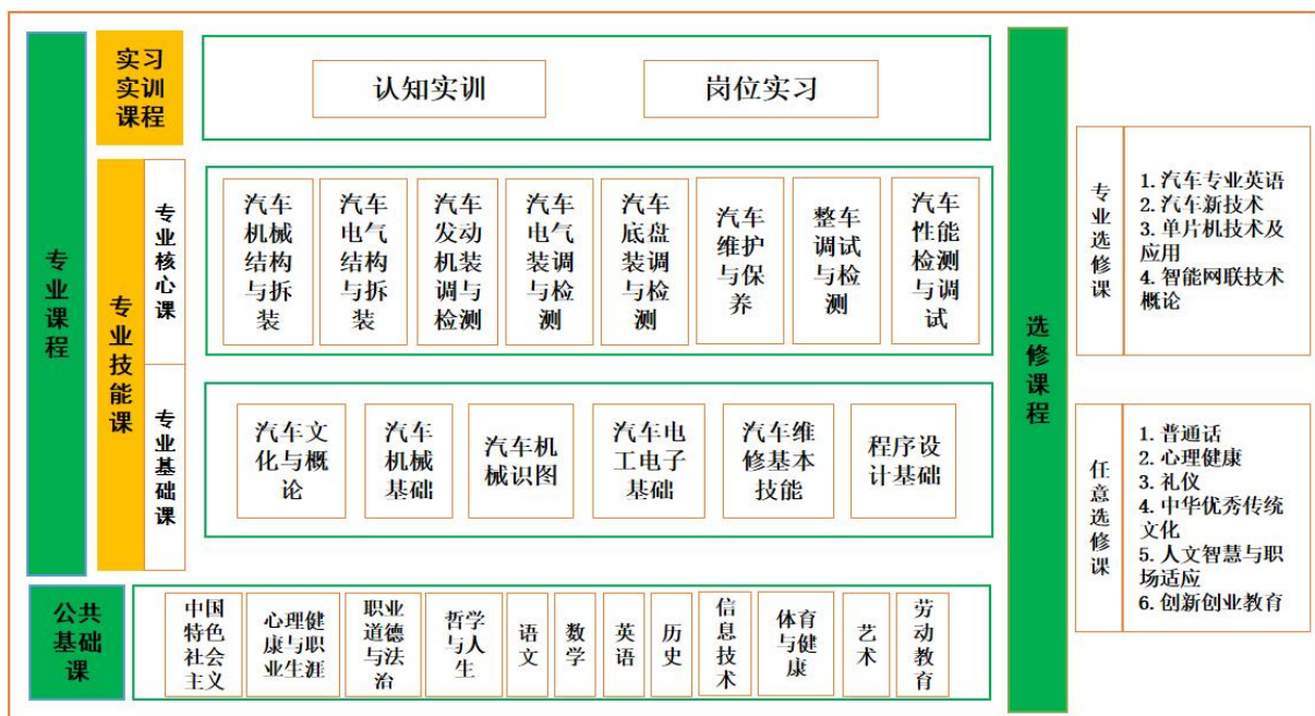
图 1 课程结构图
